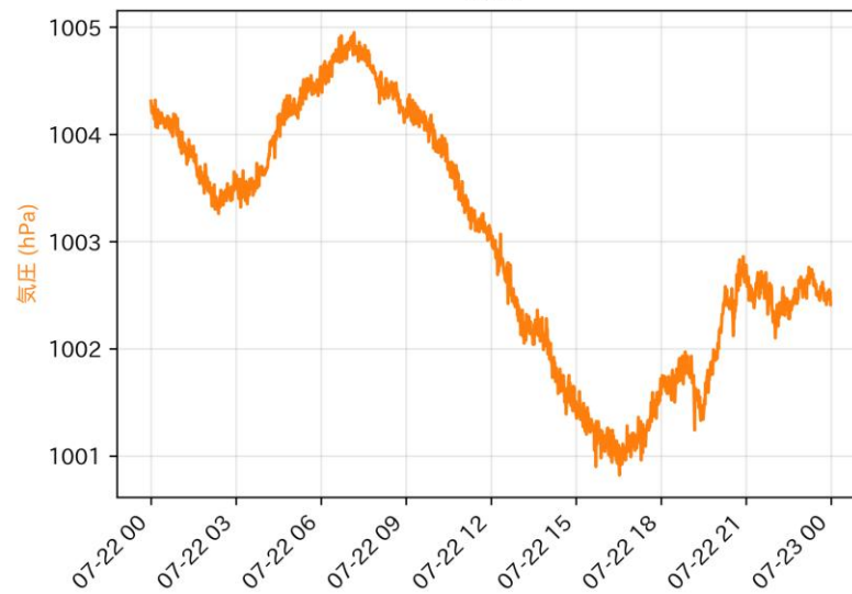
気圧
