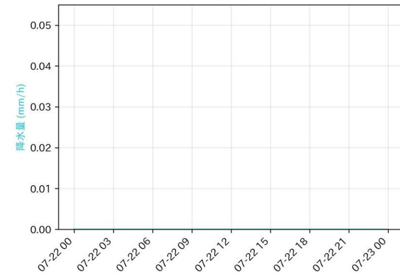
降水量
