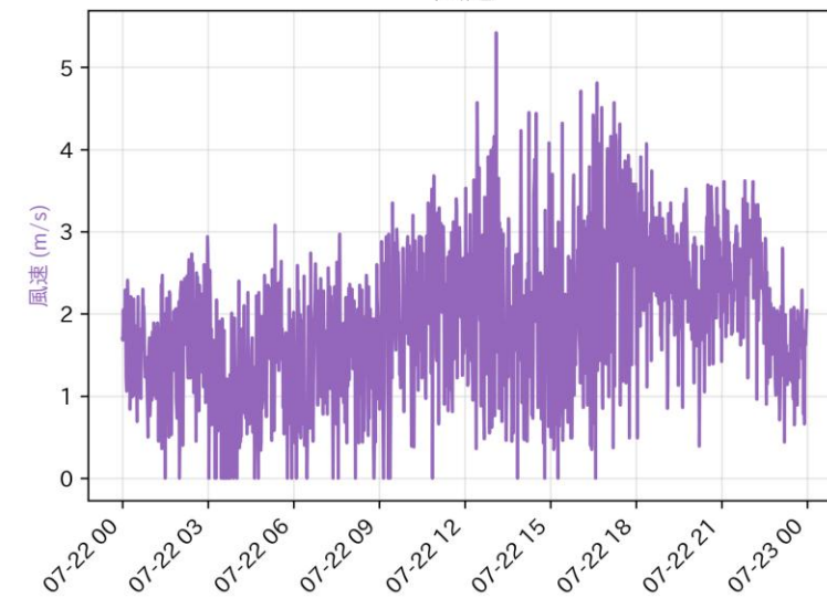
風速
